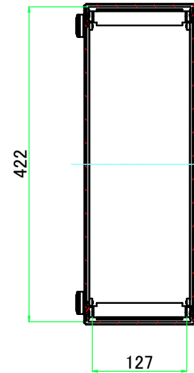
B-B ( 1 : 7 )
